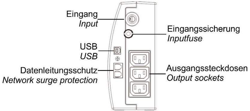
Abbildung 4: Rückansicht YUNTO 500 - 800
