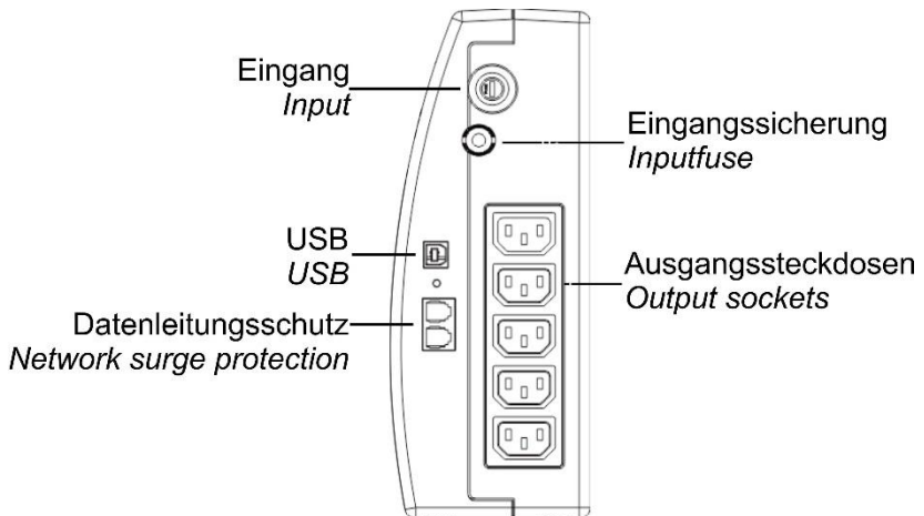
Abbildung 5: Rückansicht YUNTO 1200 - 1500
